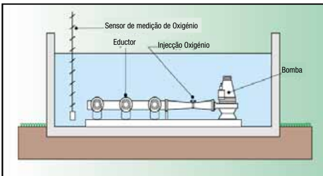
Sistema de Arejamento Halia® de instalação directa
