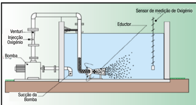
Sistema de Arejamento Halia® de instalação fixa
